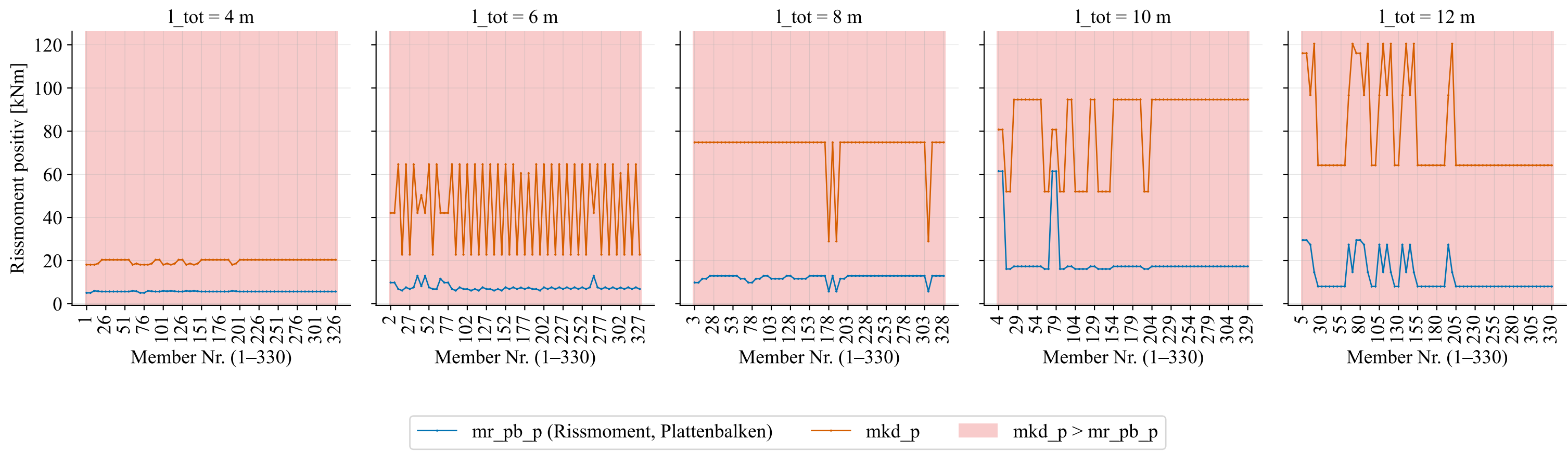
Rissmoment mr_pb_p (Plattenbalken) vs. Moment mkd_p (positive Biegung) je Member, kategorisiert nach Spannweite (Members_rc_rib_simple_V3)
